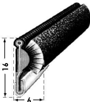
Flat flexolist (børstelist, m/metallkant)
